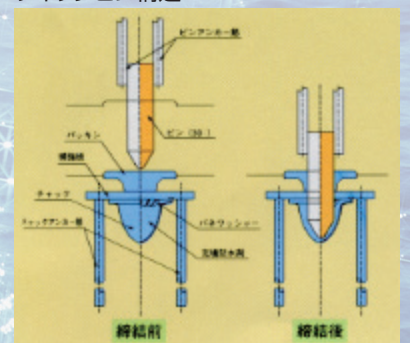
チャックピン構造
